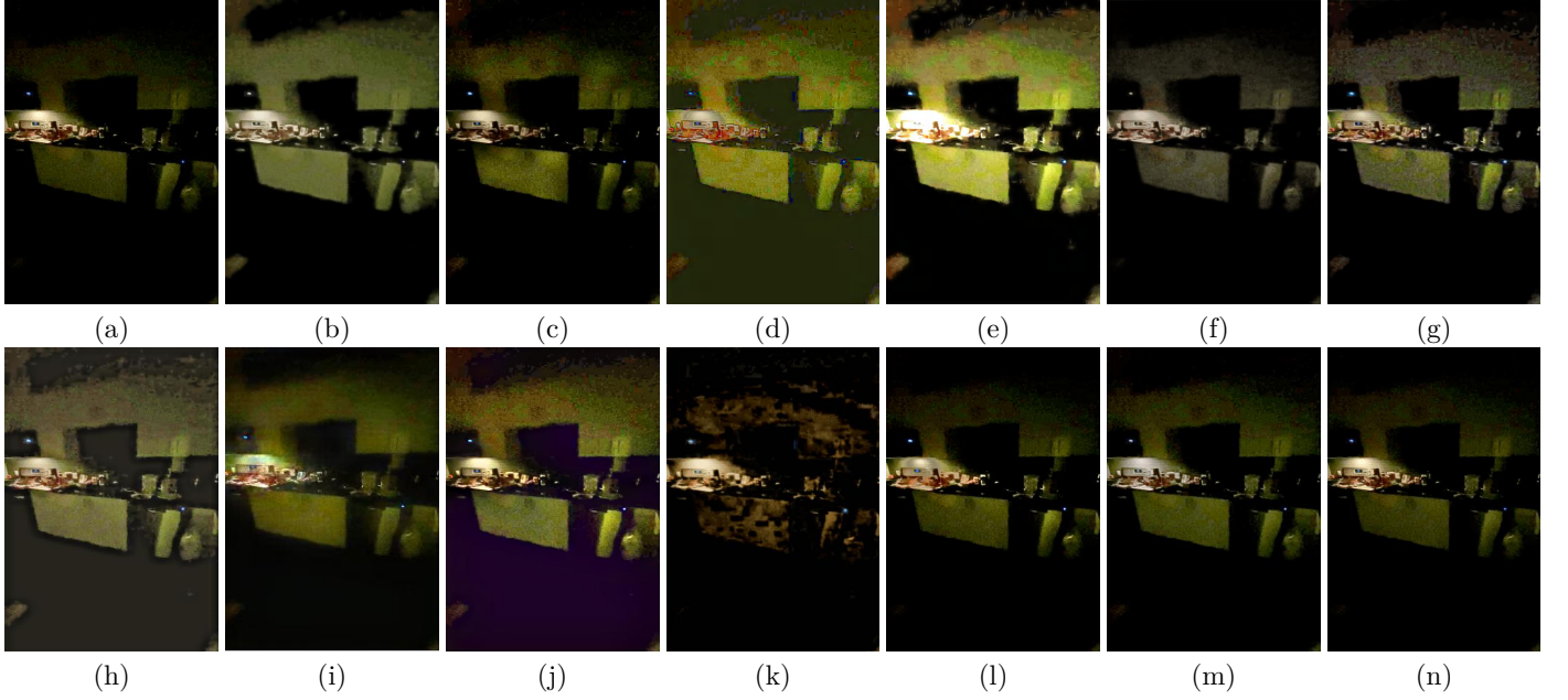
图 7. 不同方法在 LLIV-Phon-imgT 数据集取样的低照度图像上的视觉效果。(a) input. (b) LLNet [11]. (c) LightenNet [15]. (d) Retinex-Net [14]. (e) MBLLEN [13]. (f) KinD [21]. (g) KinD++ [61]. (h) TBEFN [30]. (i) DSLR [31]. (j) EnlightenGAN [36]. (k) DRBN [43]. (l) ExCNet [37]. (m) Zero-DCE [38]. (n) RRDNet [39].
