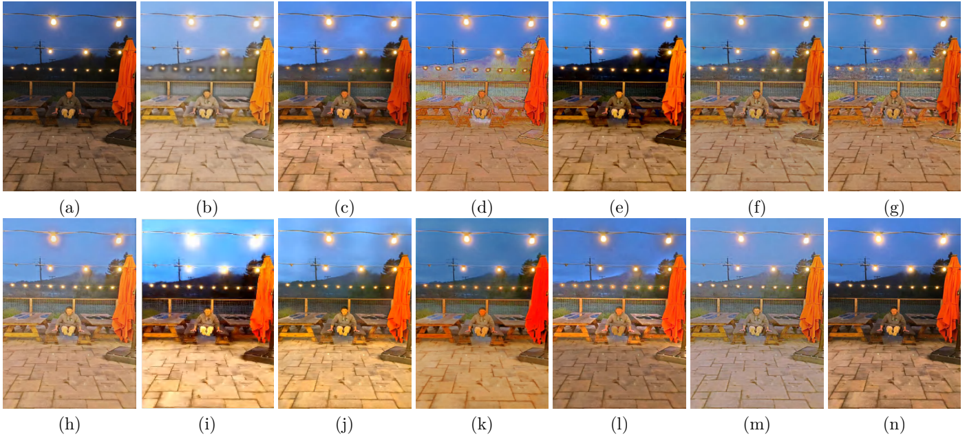
图 8. 不同方法在 LLIV-Phon-imgT 数据集取样的低照度图像上的视觉效果。(a) input. (b) LLNet [11]. (c) LightenNet [15]. (d) Retinex-Net [14]. (e) MBLLEN [13]. (f) KinD [21]. (g) KinD++ [61]. (h) TBEFN [30]. (i) DSLR [31]. (j) EnlightenGAN [36]. (k) DRBN [43]. (l) ExCNet [37]. (m) Zero-DCE [38]. (n) RRDNet [39].
