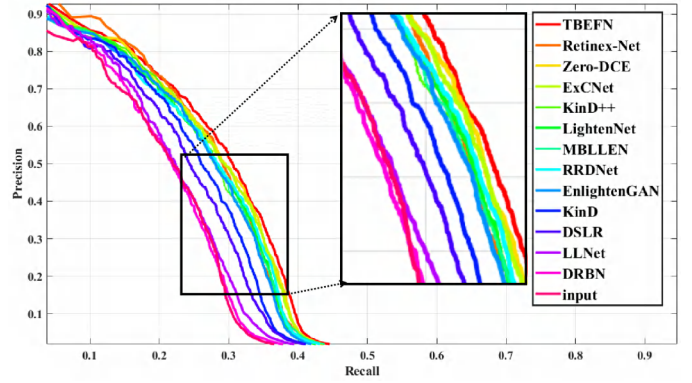
图 10. 黑暗中人脸检测的 P-R 曲线
