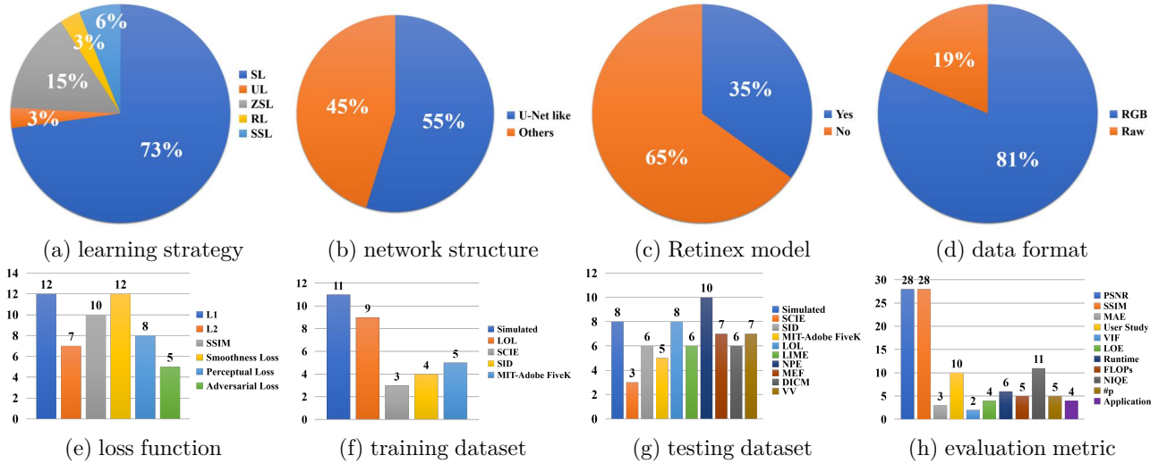
图 3. 基于深度学习的 LLIE 方法的统计分析, 包括学习策略、网络特征、Retinex 模型、数据格式、损失函数、训练数据集、测试数据集和评价指标。可放大图片查看详情。
